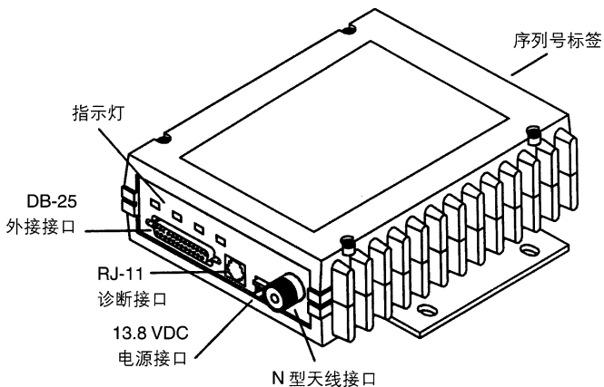
图 1 电台接口和指示灯
