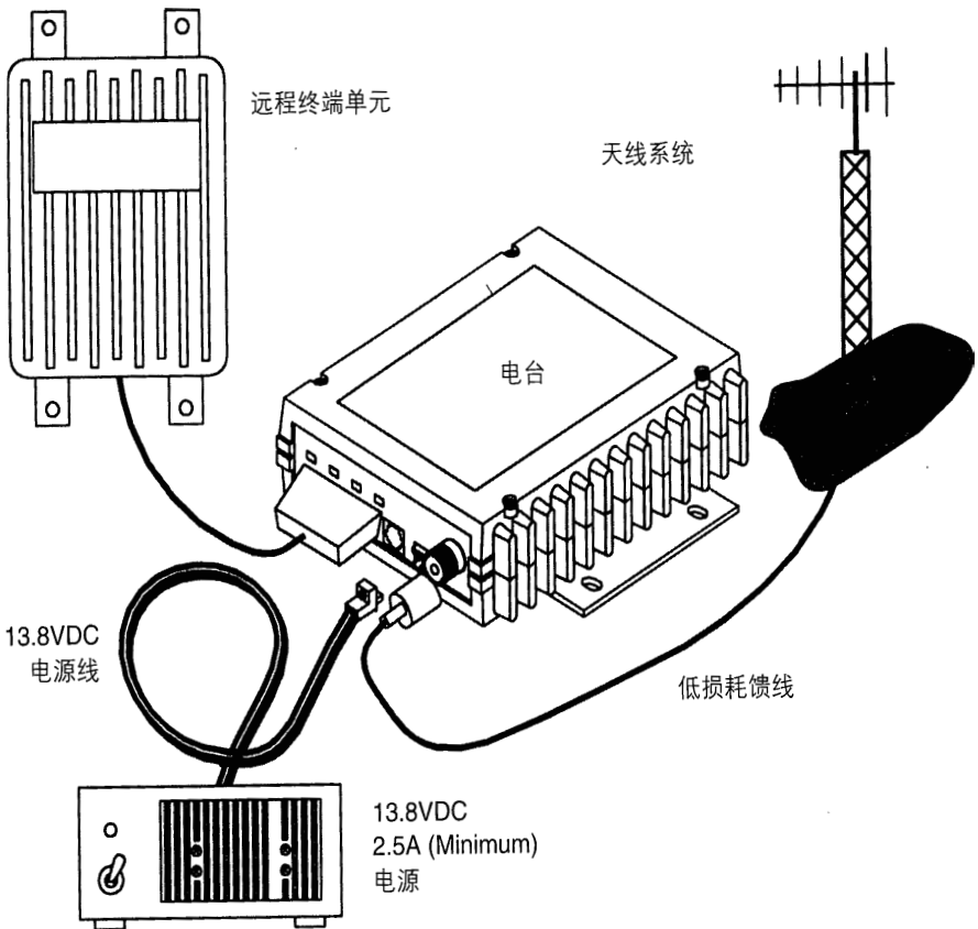
图6 典型远程站配置
