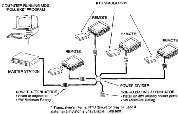
图 12 室内安装测试
