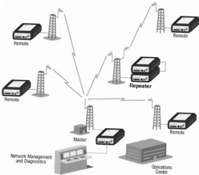
图4 典型的中转系统
