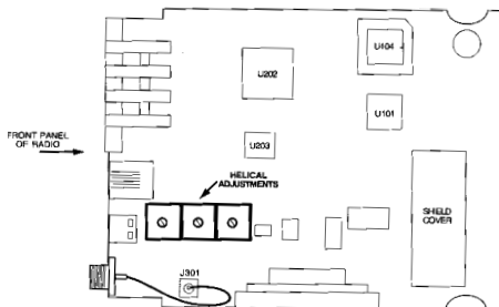
图 13 滤波器的位置
