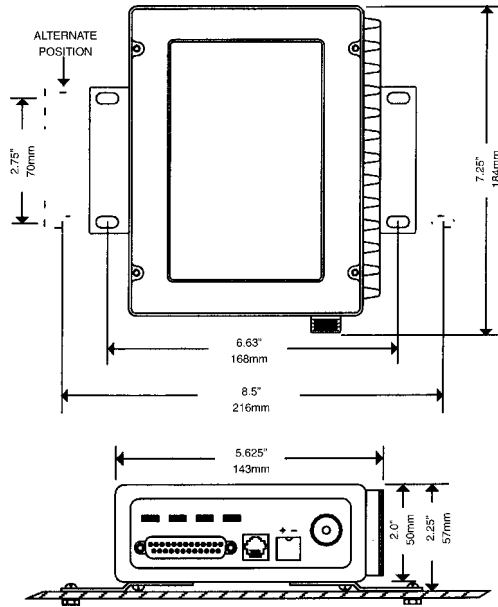
图7 电台安装尺寸
