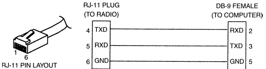
图 11 RJ-11 到 DB-9 适配连线
