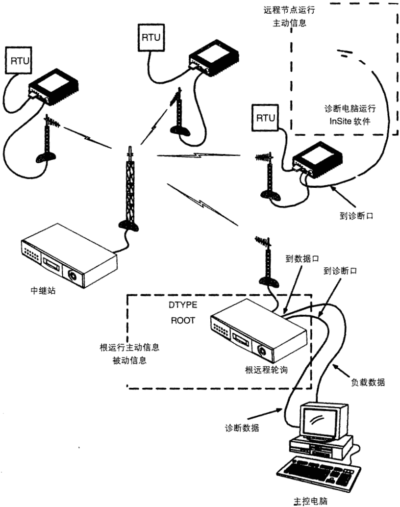
图 10 网络远程诊断设置
