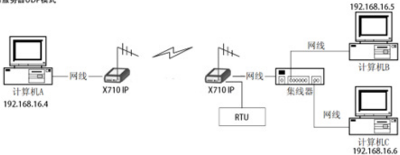
串口服务器UDP模式
