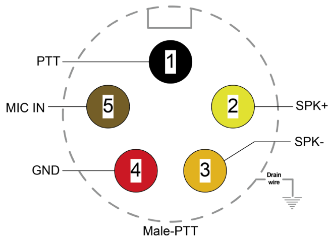
图 3 PTT 引脚说明图 (接线端)
