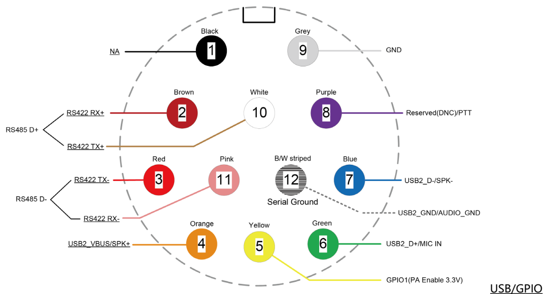
图 2 USB/GPIO 引脚说明图 (接线端)
