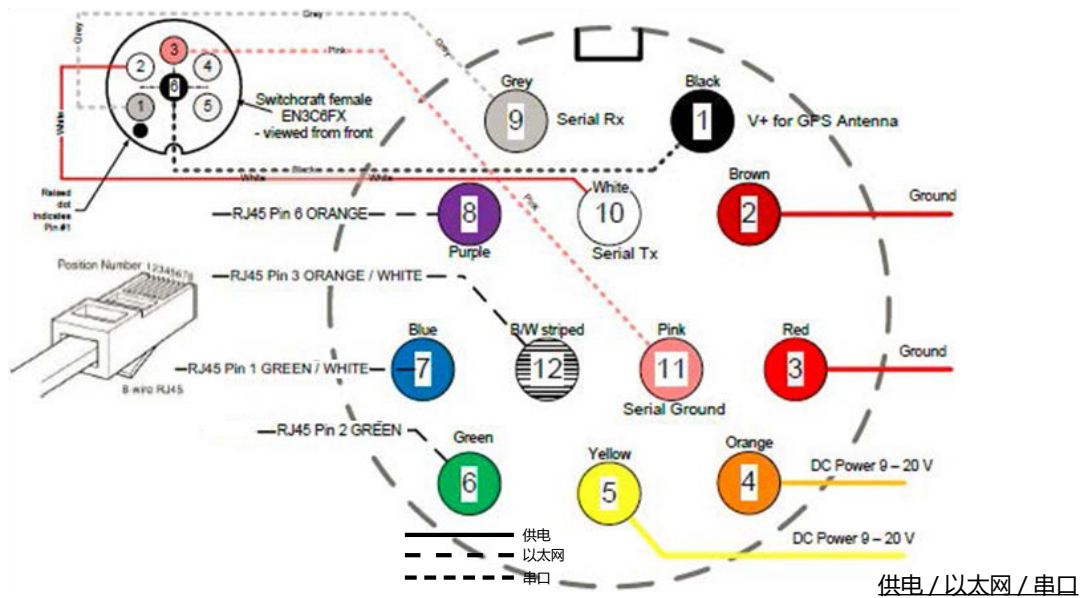
图 1 供电 (可选) / 串口 / 以太网引脚说明图 (接线端)
